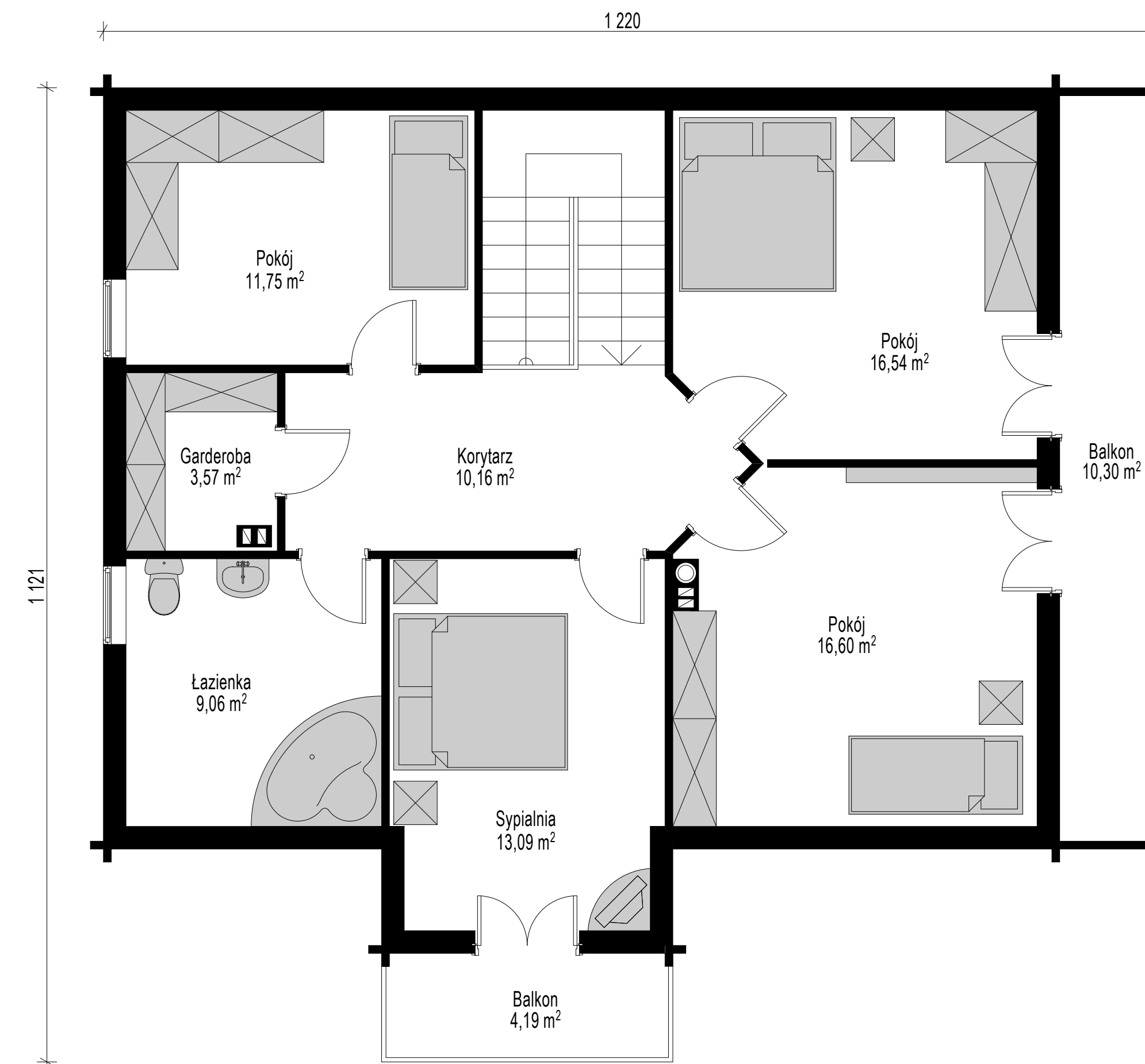
Rzut parteru pow. 80,80 m 2 + balkony pow. 14,49 m 2
