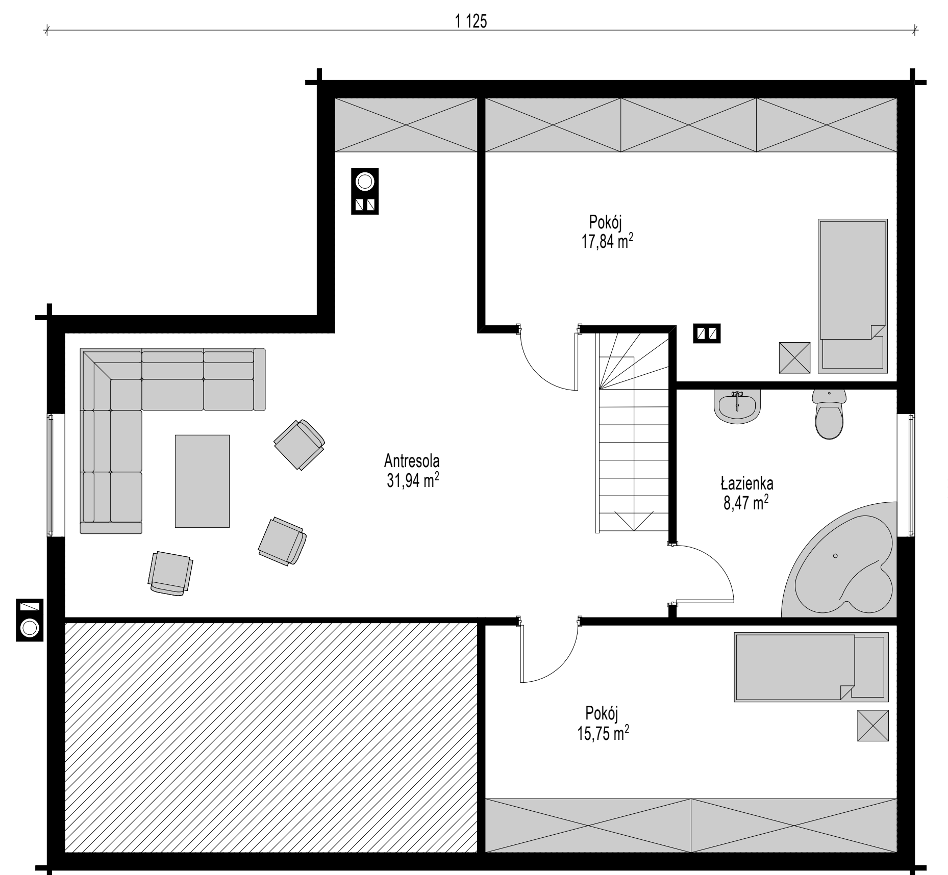
Rzut poddasza pow. 74,00 m 2
