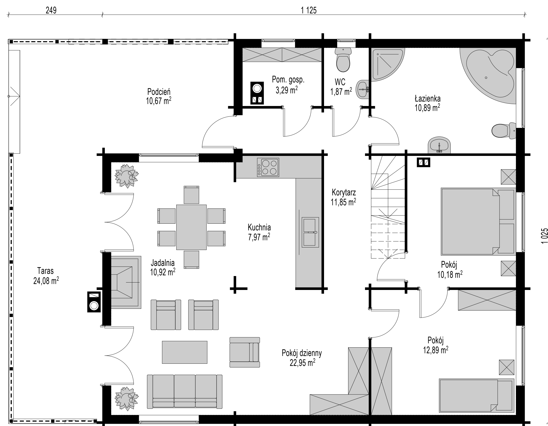
Rzut parteru pow. 92,81 m 2 + podcień pow. 10,67 m 2 + taras pow. 24,08 m 2
