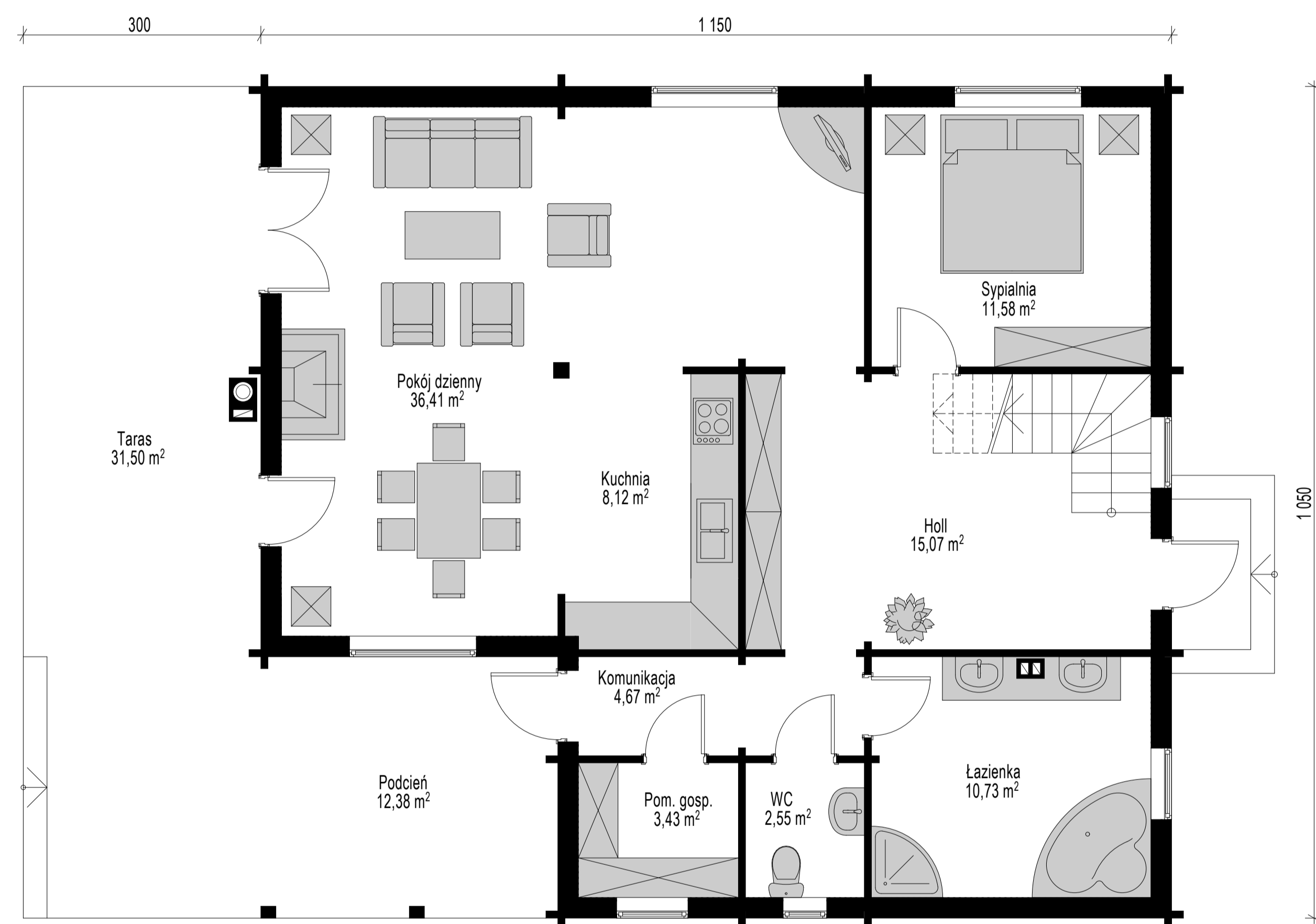
Rzut parteru pow. 92,56 m 2 + podcień pow. 12,38 m 2 + taras pow. 31,50 m 2
