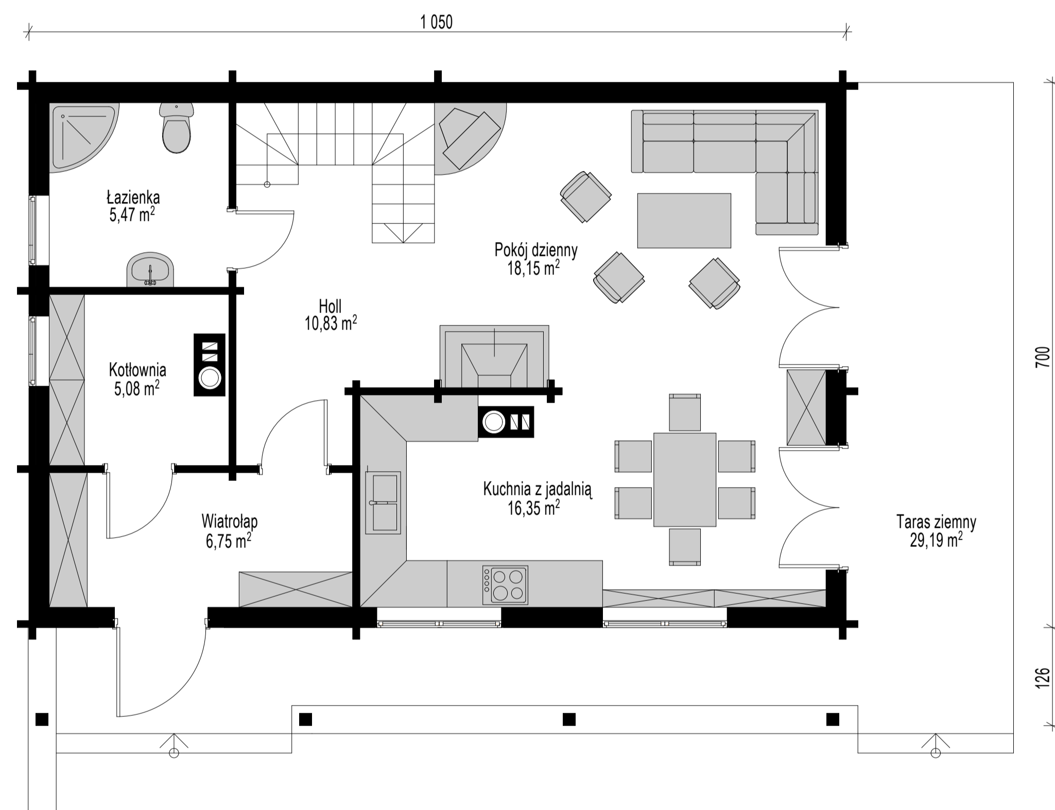
Rzut parteru pow. 62,63 m 2 + taras ziemny pow. 29,19 m 2
