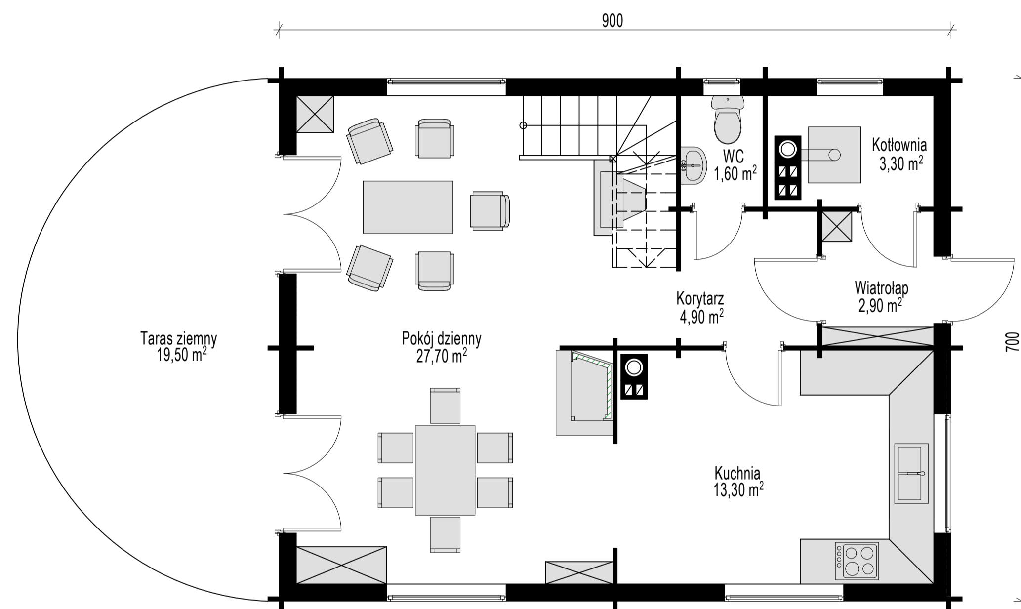
DREWEX Rzut parteru pow. 53,70 m 2 + taras 19,50 m 2
