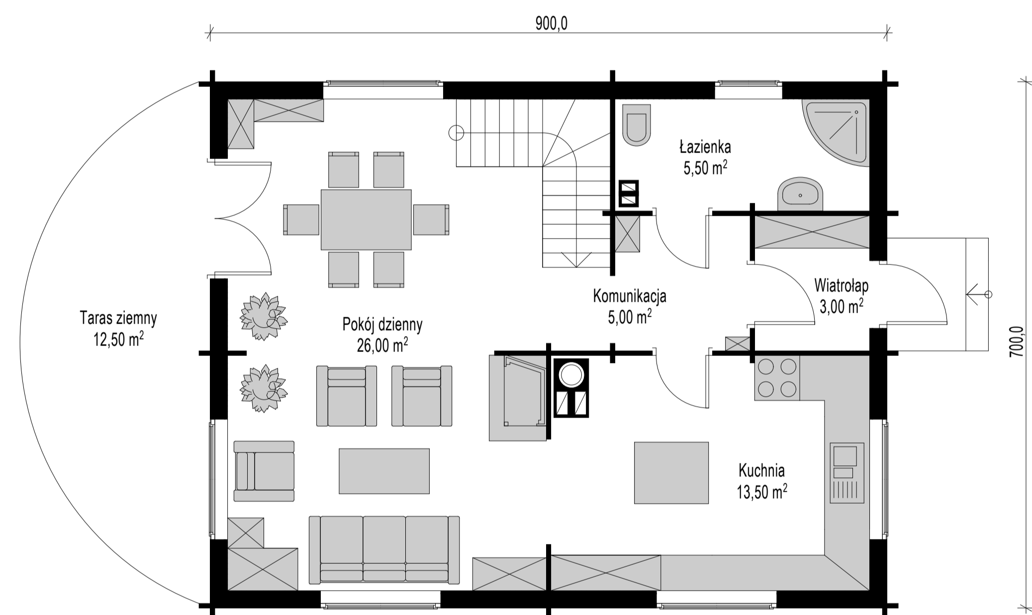
DREWNEK Rzut parteru pow. 53,00 m 2 + taras ziemny pow. 12,50 m 2
