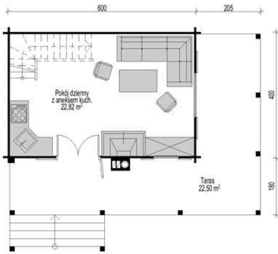
Rzut parteru pow. 22,82 m 2 + taras pow. 22,50 m 2
